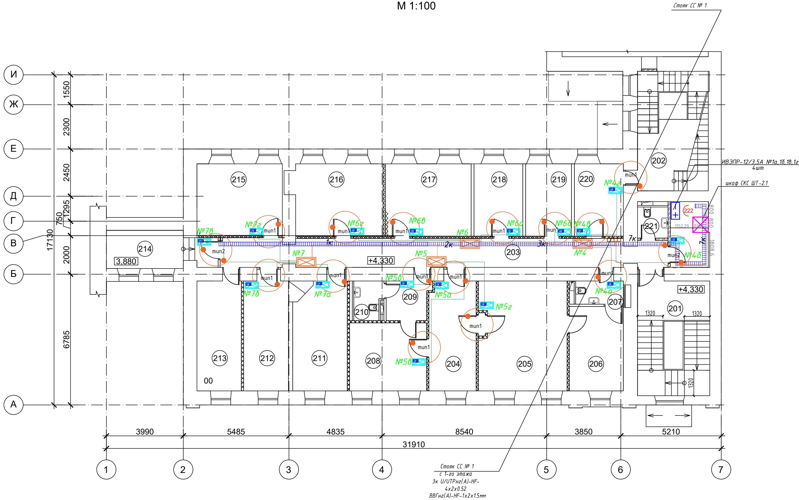
Схема расположения гильз d=50мм в перекрытиях
