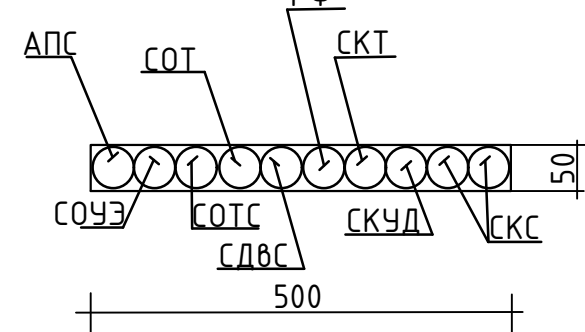
Схема расположения гильз d=50мм в перекрытиях
