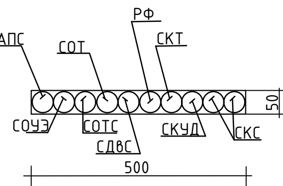
Схема расположения гильз d=50мм в перекрытиях
